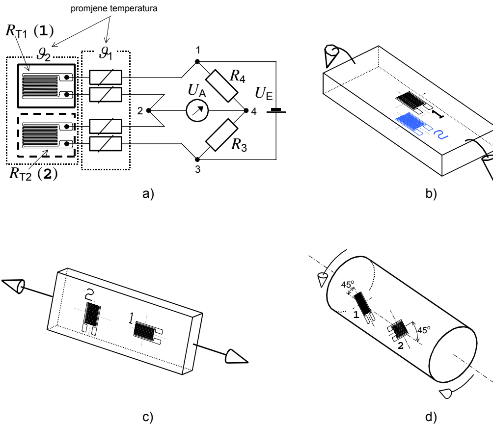
Slika 4.8. Temperaturna kompenzacija na mjernom mjestu pri poznatom stanju napreznja (polumost).
