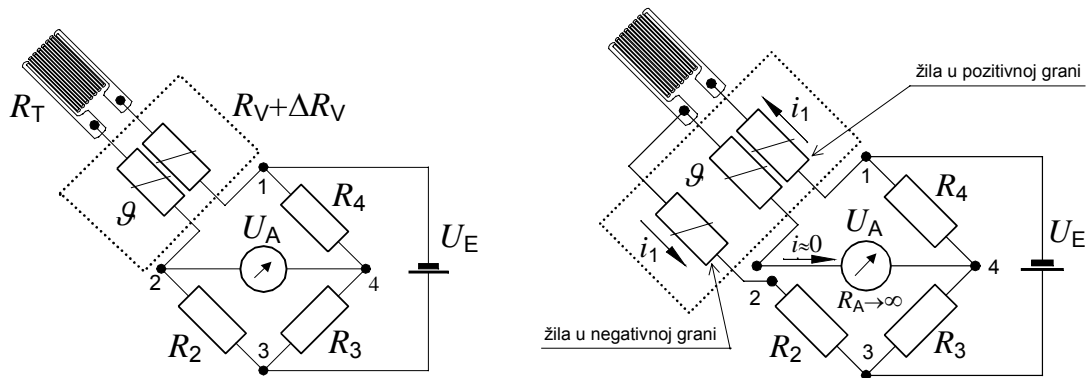
Slika 4.7. Temperaturna kompenzacija priključnih vodova (četvrtmost).
