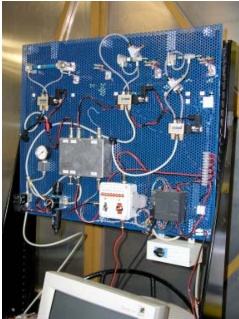
Elektropneumatički didaktički stol.
